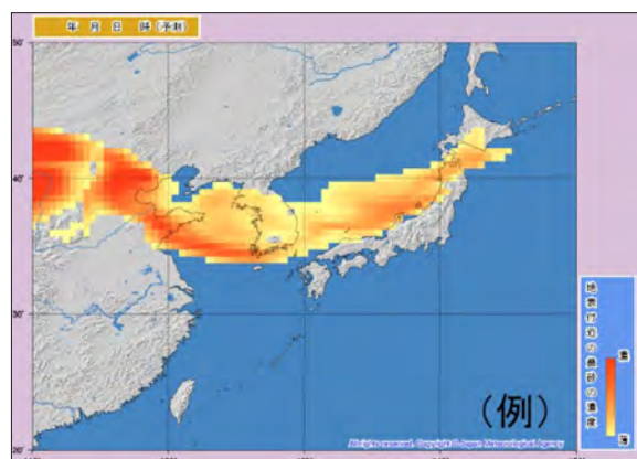
黄砂解析予測図（日本域）の例 （地表付近の黄砂の濃度の分布図）
