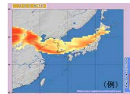
黄砂解析予測図の例
